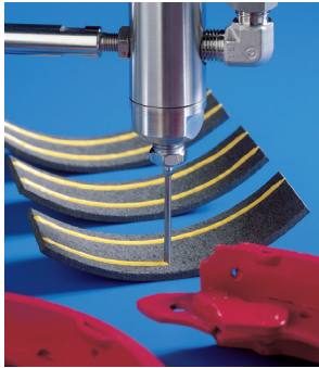
Fren pabucu balatalarına yapısal yapıştırıcı uygulaması.
